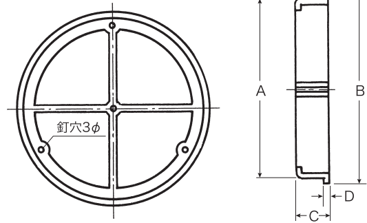
■ 寸法図
