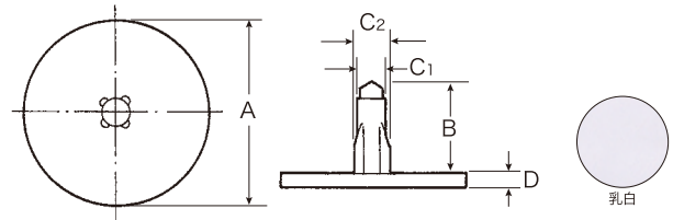
■寸法図
